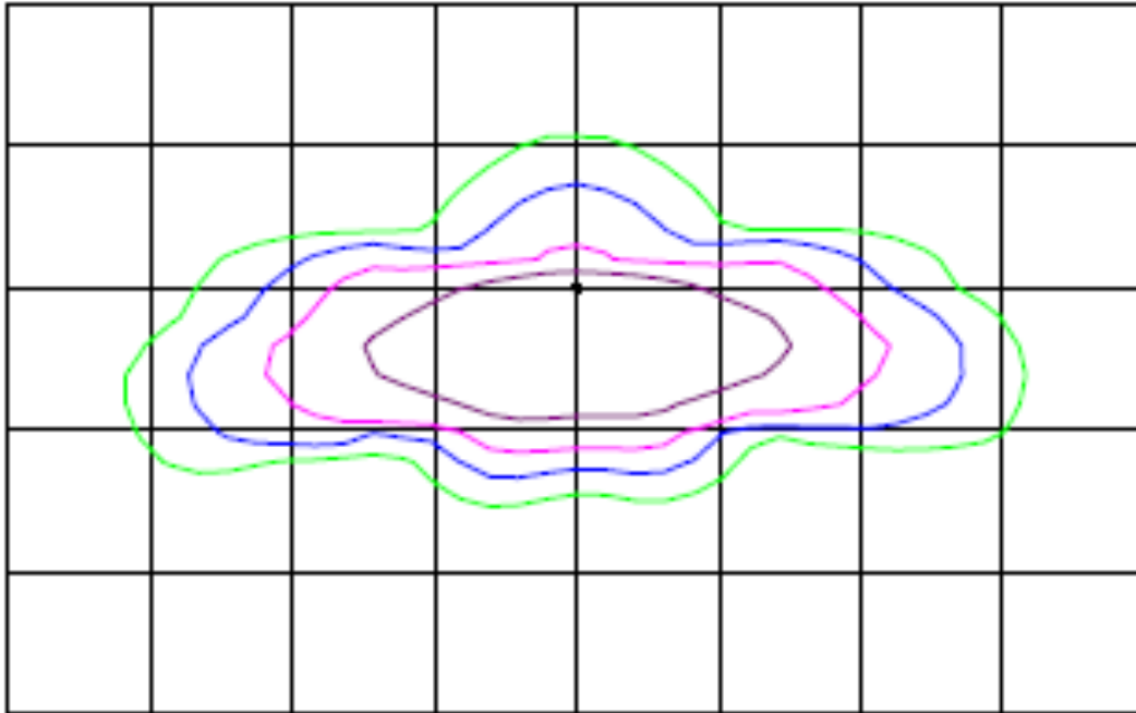
Type II: Roadway
